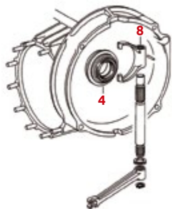
Cambio tipo 915 (1972 - 1986)
