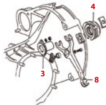
Cambio tipo 915 (1972 - 1986)
