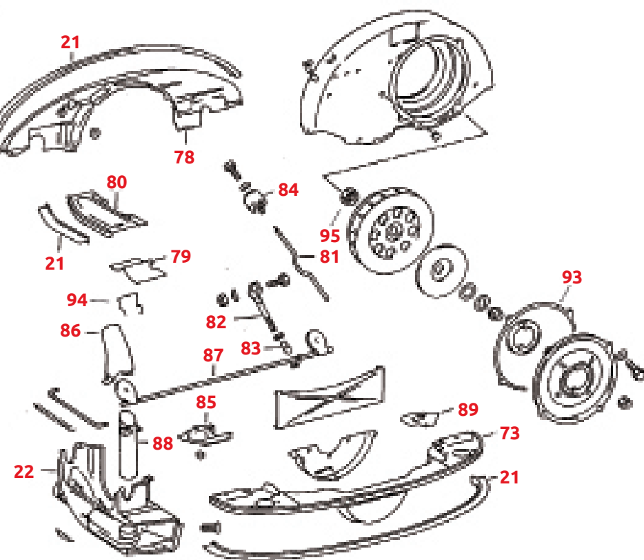
LAMIERE MOTORE
